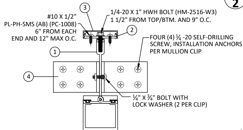
B 2 HORIZONTAL SECTION METAL STUD MULLION CLIP
